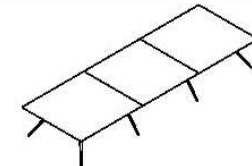
LS-ML3612W/G W3600×D1200×H750 LS-ML4816W/G W4800×D1600×H750
