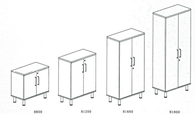
Two Wooden Door Cupboard M6B-2WDC-08 W800×D420×H800 M6B-2WDC-12 W800×D420×H1200 M6B-2WDC-16 W800×D420×H1600 M6B-2WDC-20 W800×D420×H2000
