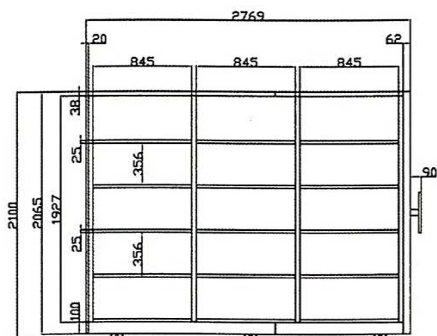
Rail Position Drawings 路軌位置圖
